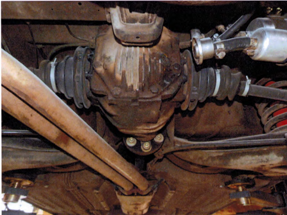
Foto 15 zeigt das Differenzial Ölverlust frei
