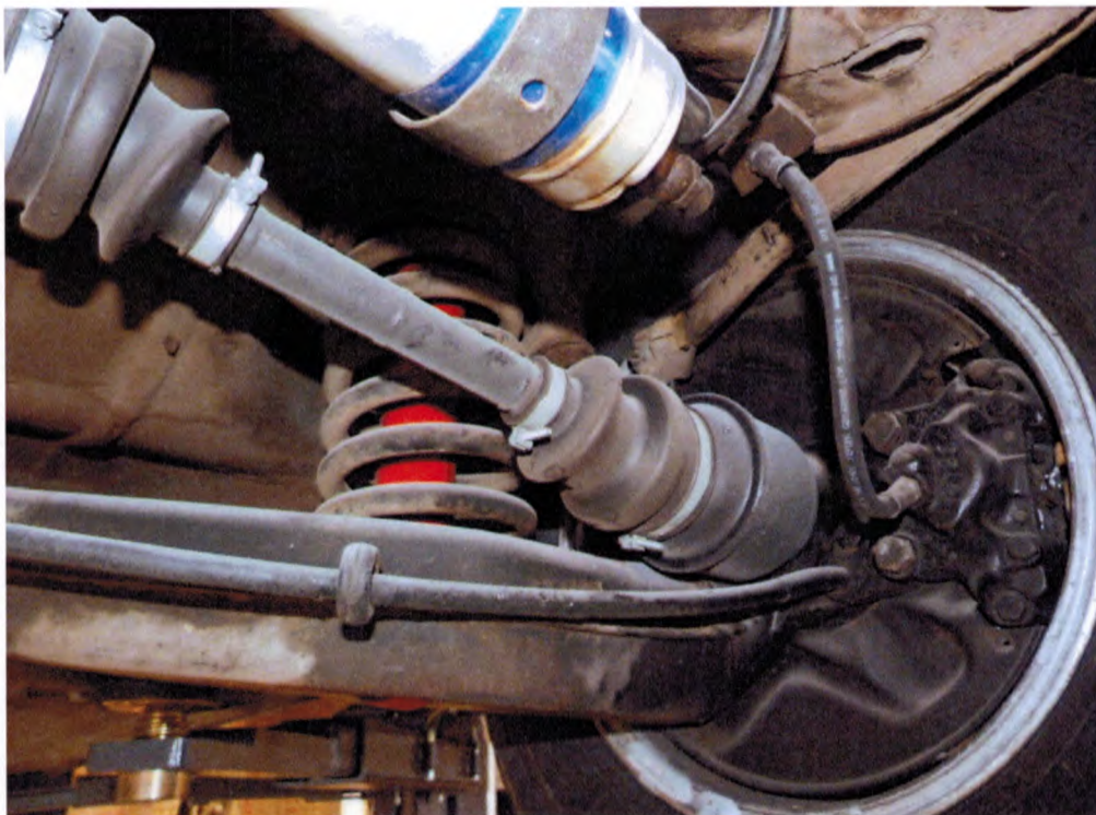
Foto 14 zeigt Hinterachse mit Querlenker und Antriebswelle
